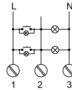
instalacja 3-przewodowa
